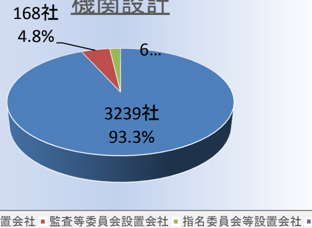
機関設計
